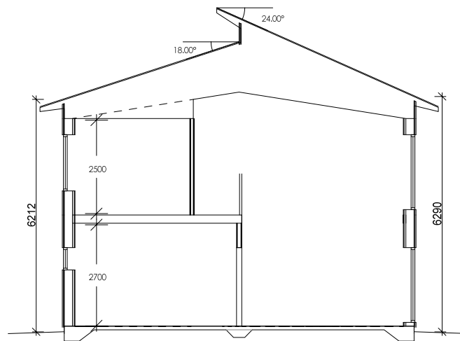
SEKTION B-B
