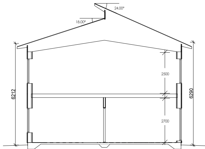
SEKTION A-A
