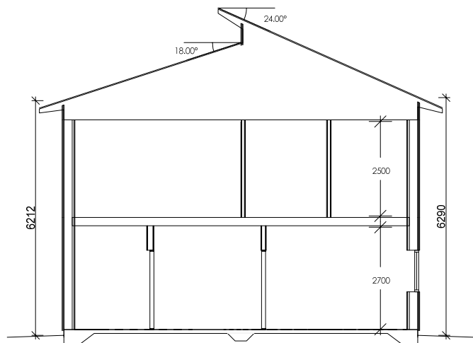
SEKTION C-C
