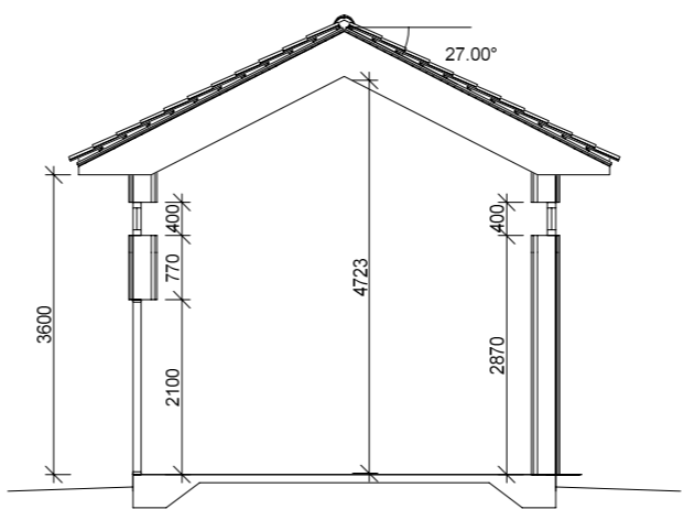
SEKTION B-B
